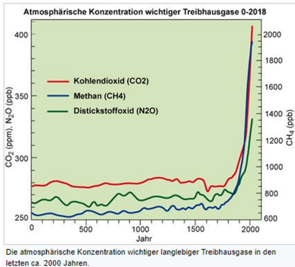
Abbildung 1 - Konzentration von Treibhausgasen ( wiki.bildungsserver.de )
